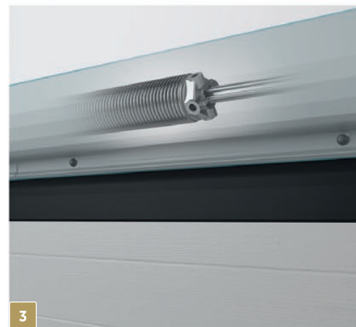
Integruotas veleno ir spyruoklės dangtis
