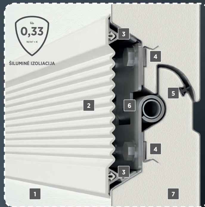
„PRIME“, „UniTherm“ garažo vartai
