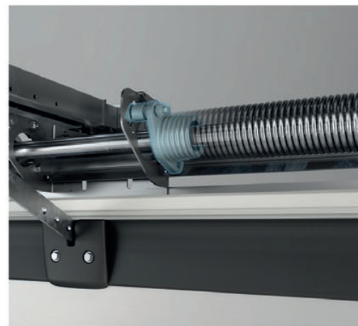
Integruotas spyruoklės nutraukimo saugos įtaisas
